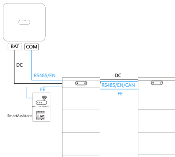
Abbildung 2-10 Anschließen der ESSs an den Wechselrichter (1)
