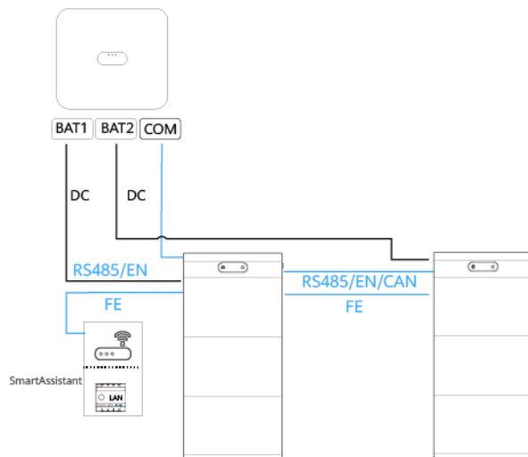
Abbildung 2-11 Anschließen der ESSs an den Wechselrichter (2)
